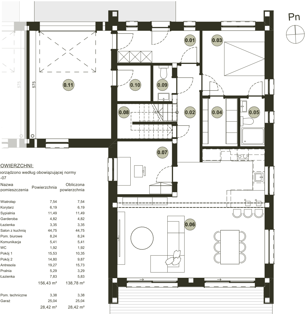
Rzut Parteru
