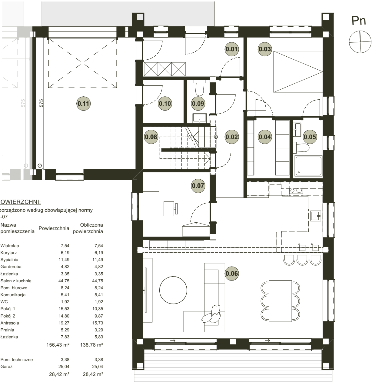
Rzut Parteru
